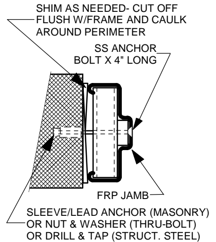
SECTION THRU JAMB
